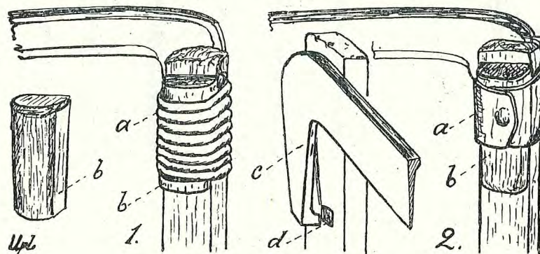
Fig. 4. Liens fastsättande vid orvet.
