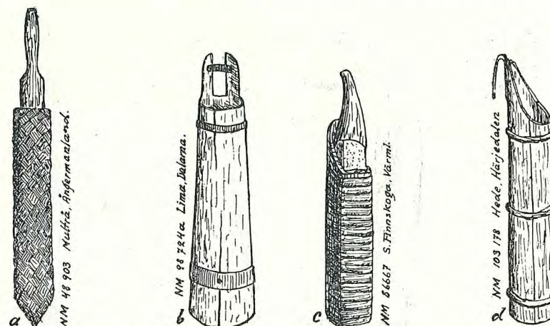
Fig. 7. Brynfodral och brynbyttor.
